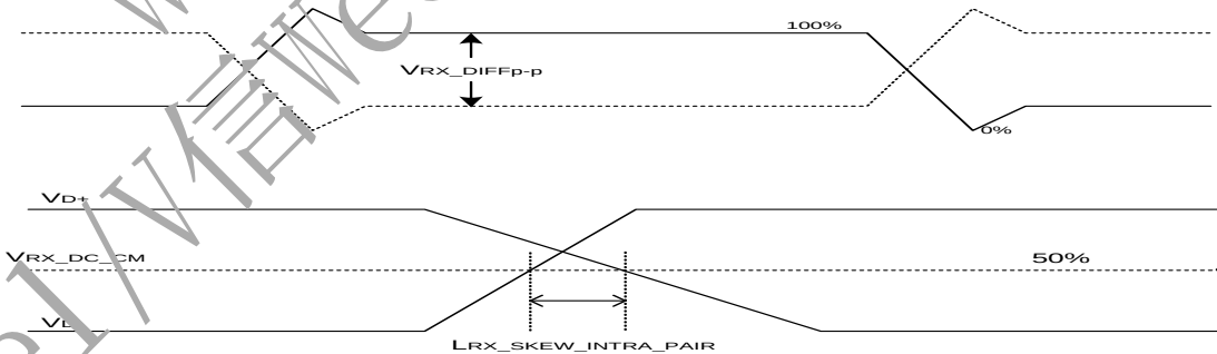
Figure 14. VRX-DIFFp-p & LFX_SKEW_INTRA_PAIR
